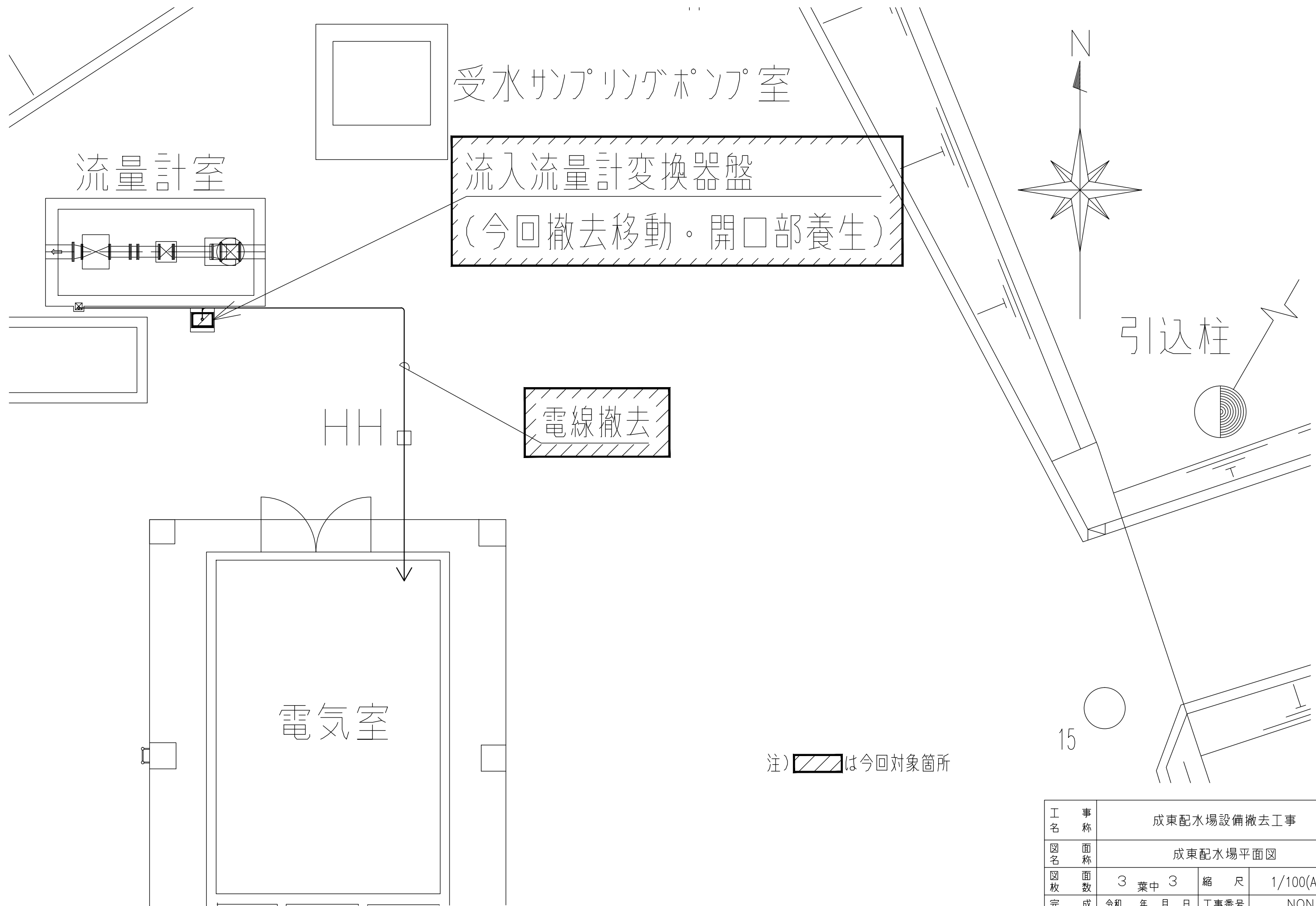
成東配水場平面図
