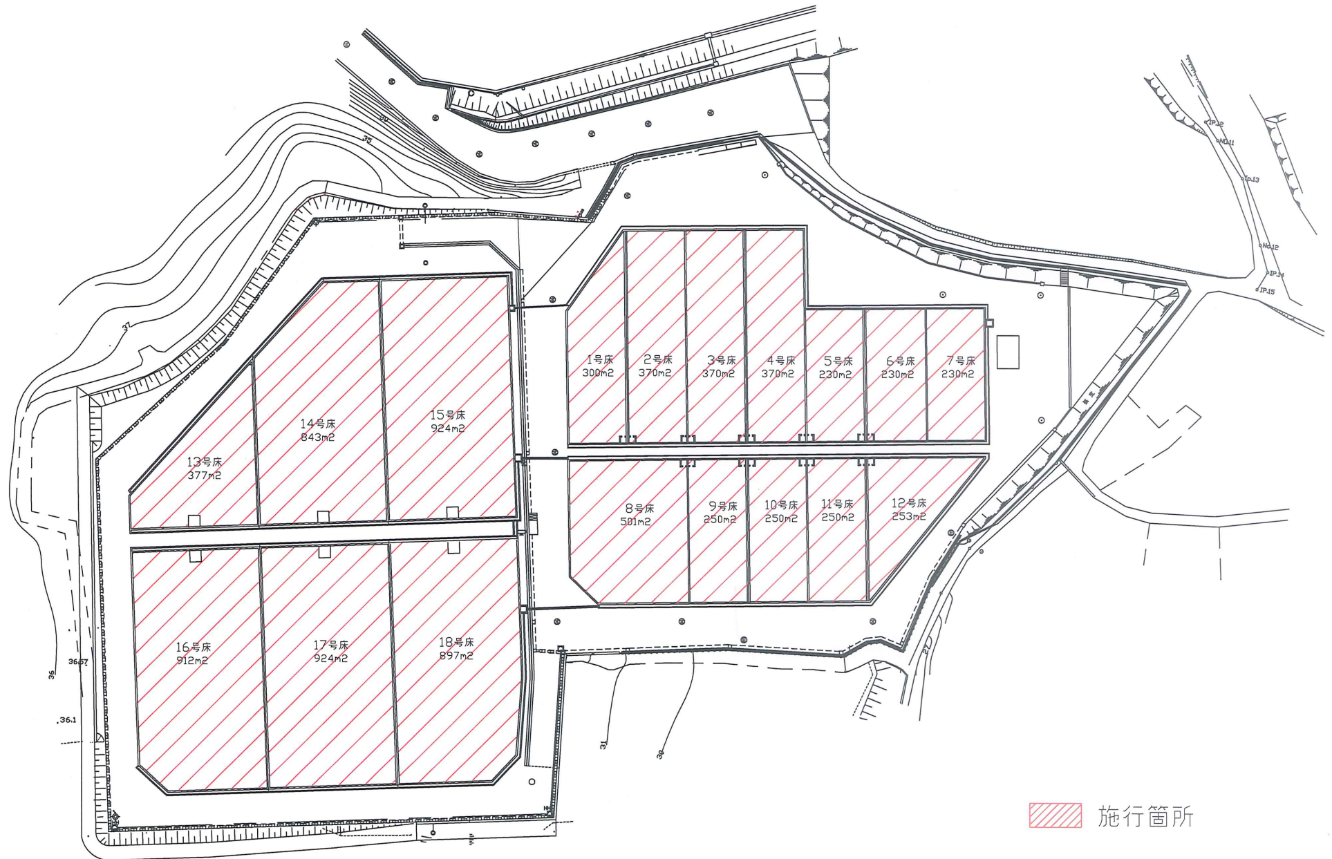
光天日乾燥場平面図
