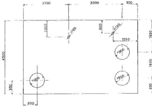
頂版開口位置図
