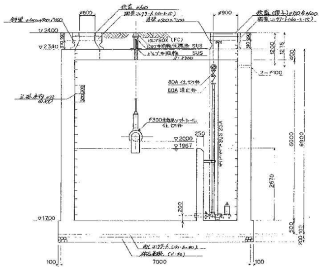
A-A断面
