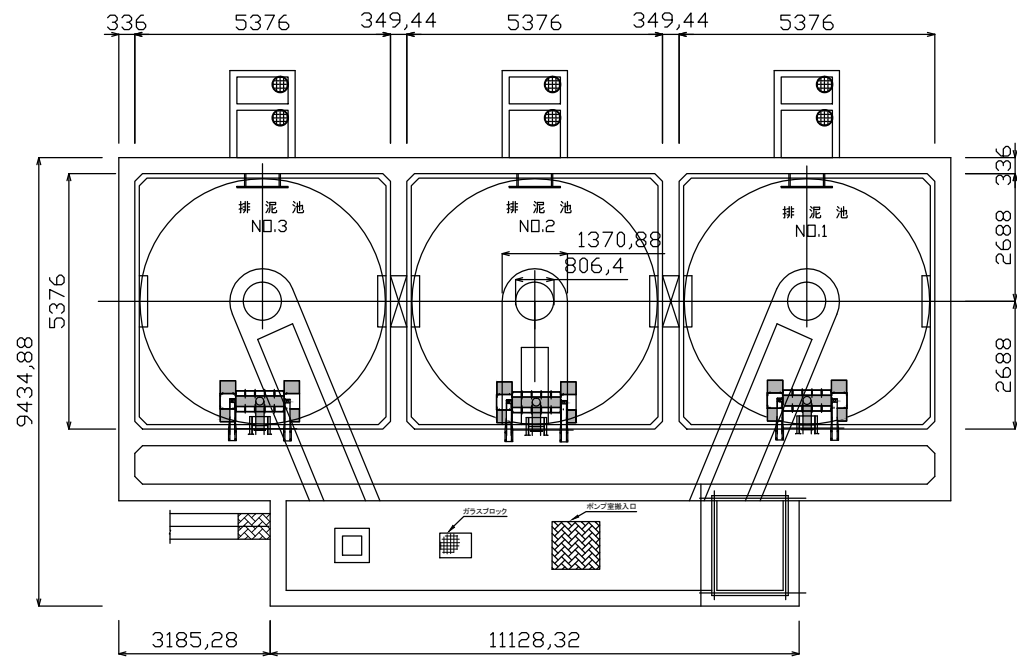
排泥池平面図
