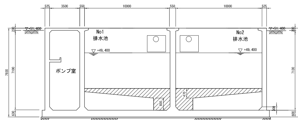
A—A' 断面図
