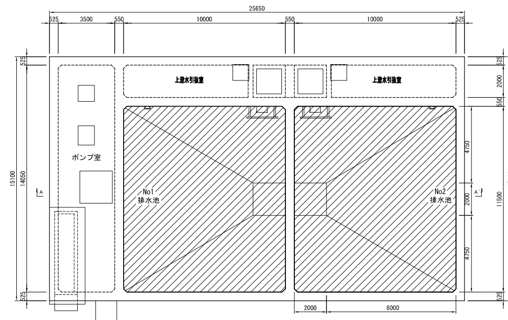
排水池平面図
