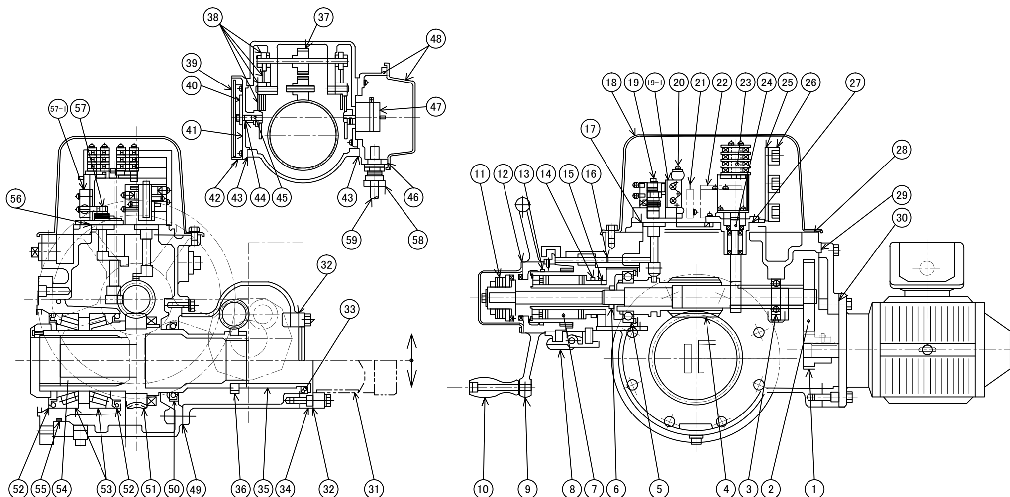
バルブコントロール詳細図 (LTKD-05)
