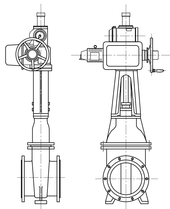
電動仕切弁外形図 (φ300外ネジ式)
