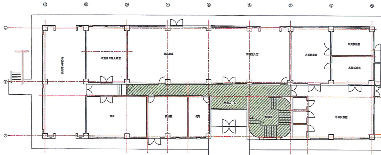
1階 平面図
